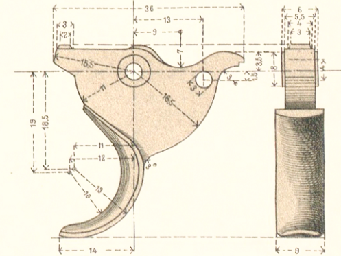
SCHALTER. 6. POUSSEUR.
