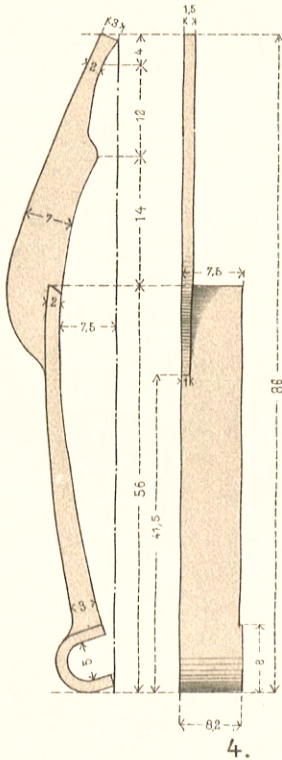
4. SCHLAFGEFEDER. RESSORT DE PERCUSSION.
