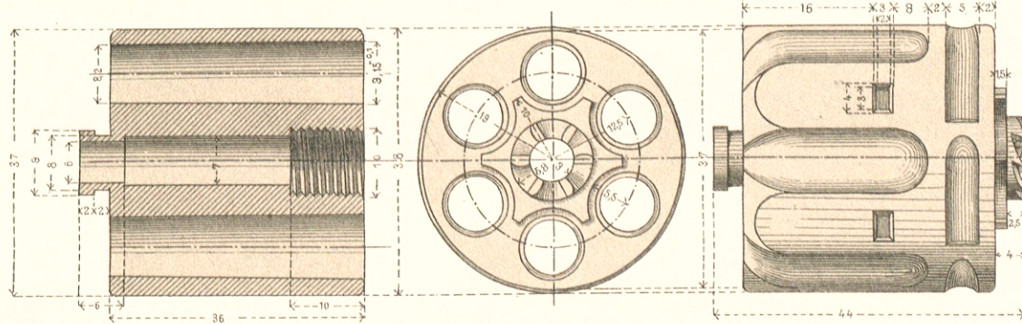
S. SCHALTRAD. ROUE À ROCHET.
