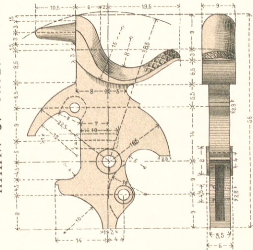
HAHN. 8. CHIEN.
