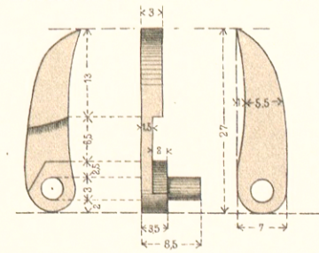
SCHALTER. 6. POUSSEUR.
